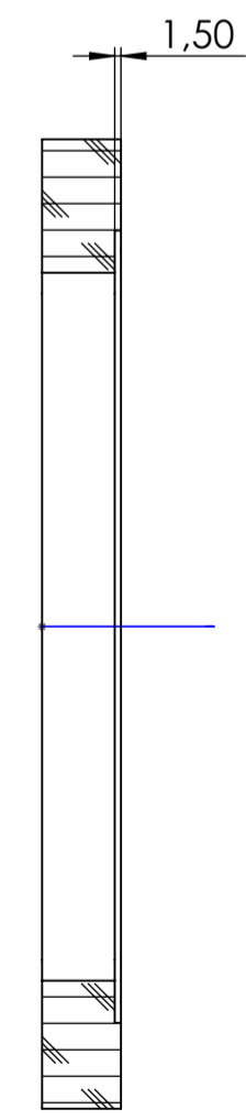
SCHNITT B-B
