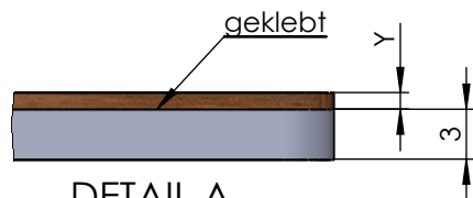
DETAIL A MAßSTAB 2 : 1
