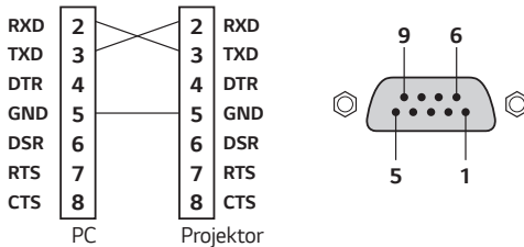
Abbildung 1: RS-232-Verbindungsdiagramm
